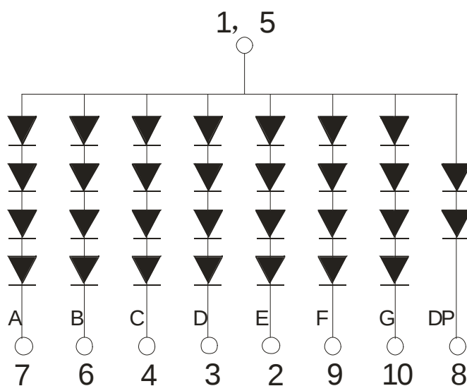
数码管显示及引脚位置图
